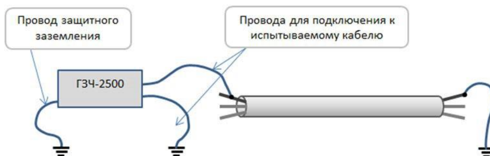
Рисунок 3. Трассировка кабеля.
